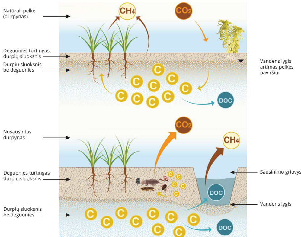
1 pav. Anglies ciklas natūraliose pelkėse ir sausinimo pažeistuose durpynuose. Adaptuota pagal Jan Peters, Michaelio Zukovo gamtos apsaugos fondas (Vokietija). Ilustracijos autorius Nieves Lopez Izquierdo (2017) ( https://www.grida.no/resources/12532 ).
