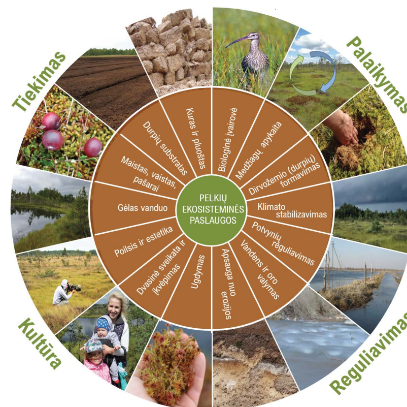
4 pav. Pelkių ekosistemines paslaugas – pelkių mums teikiama nauda. Adaptuota pagal Millennium Ecosystem Assessment, 2005. Ilustracijos autorė Jūratė Sendžikaitė
